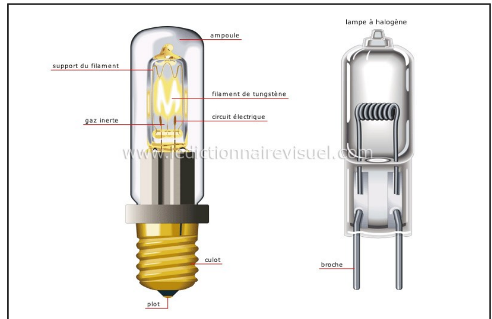
Lampe à incandescence
