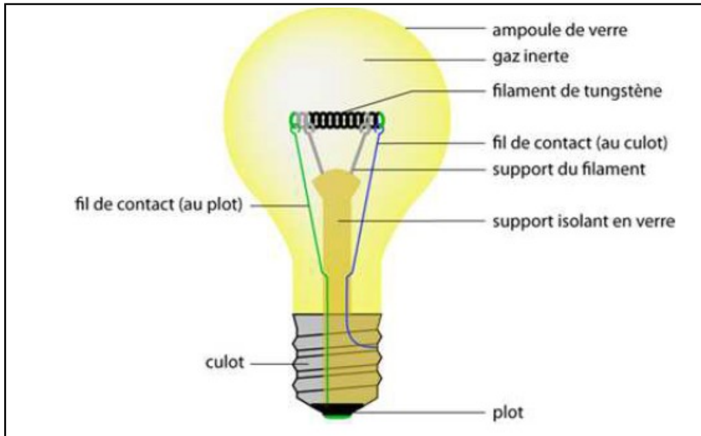
Lampe à incandescence
